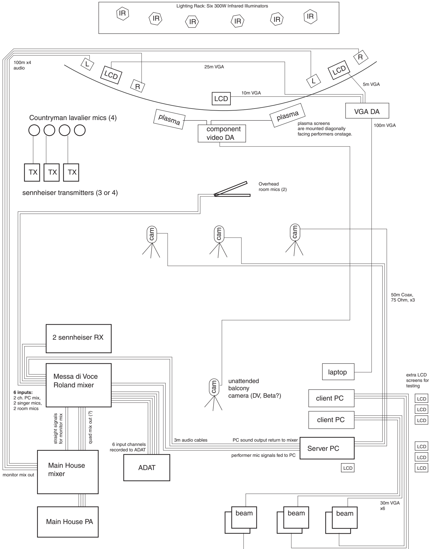
Messa di Voce: Lighting/Sound/Video Wiring Diagram
